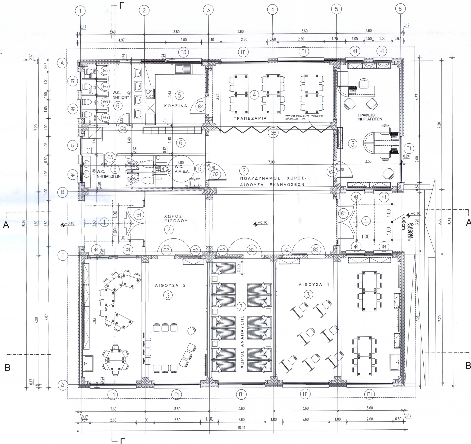
ΚΑΤΟΨΗ ΙΣΟΓΕΙΟΥ ΕΜΒΑΔΟΝ ΙΣΟΓΕΙΟΥ : 18,34 X 18,34 = 336,35Μ2
